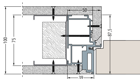
Telaio su parete in cartongesso con due lastre - Spessore parete finita 100 mm
