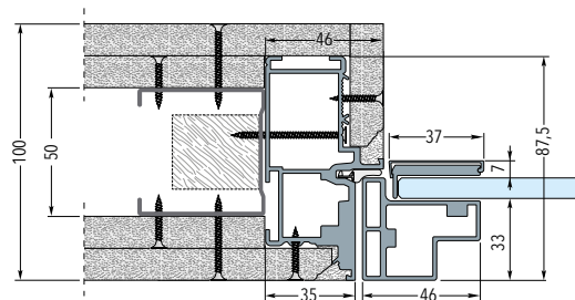
Telaio su parete in cartongesso con due lastre - Spessore parete finita 125/150 mm
