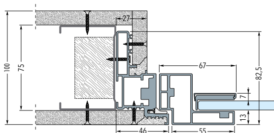
Telaio su parete in cartongesso con due lastre - Spessore parete finita 100 mm
