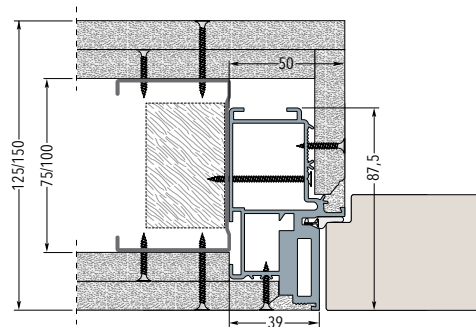
Telaio su parete in cartongesso con due lastre - Spessore parete finita 125/150 mm
