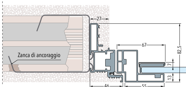
Telaio su parete in cartongesso con una lastra - Spessore parete finita 100 mm
