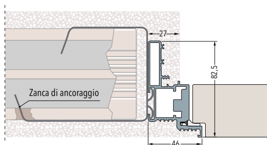
Telaio su parete per intonaco
