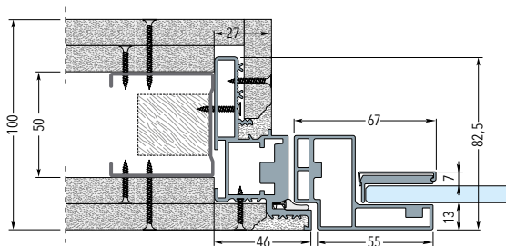
Telaio su parete in cartongesso con due lastre - Spessore parete finita 125/150 mm
