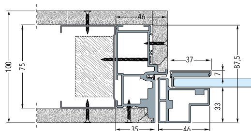
Telaio su parete in cartongesso con due lastre - Spessore parete finita 100 mm
