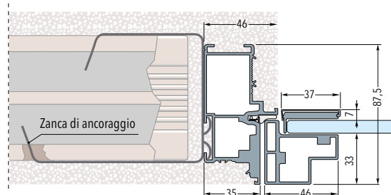
Telaio su parete in cartongesso con una lastra - Spessore parete finita 100 mm
