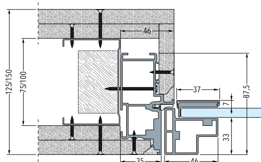
Telaio su parete in cartongesso con due lastre - Spessore parete finita 125/150 mm
