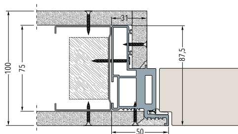
Telaio su parete in cartongesso con due lastre - Spessore parete finita 100 mm
