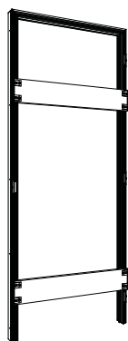
TELAIO IN ALLUMINIO PER PORTA ECLISSE SYNTESIS® BATTENTE VETRO
