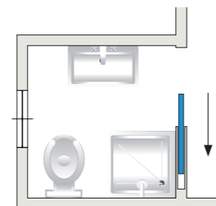
SOLUCIÓN CON SISTEMA ECLISSE EWOLUTO CORREDERO
